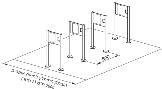
* כל המידות בשרטוטים הם במ"מ
